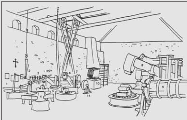
Hamernická dílna z r. 1505. 1 – manipulační stůl; 2 – váhy na železo; 3 – nářadí; 4 – kovadlina; 5 – zavěšená sedačka; 6 – „švanchamr“; 7 – transmisií převod na setrvačnicková kola s valem stlačujícím chvosty hamrů; 8 – bočně nadhazovací hamr; 9 – val stáhnutý zděřemi, osazený litinovým kroužkem s nadhazovacími palci; 10 – výheň; 11 – brus
